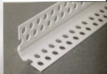
PARASPIGOLO FORATO IN PVC AD ANGOLO VARIABILE PVC MORBIDO DIM.25x25mm Codice: NAF11006MR
