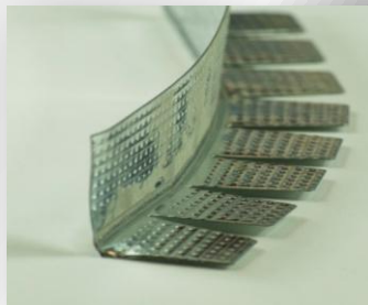
ANGOLARE FLESSIBILE IN LAMIERA ZINCATA PER COLONNE IN CARTONGESSO DIM. 30x30mm DA ML 3,0 Codice: NAF13003G
