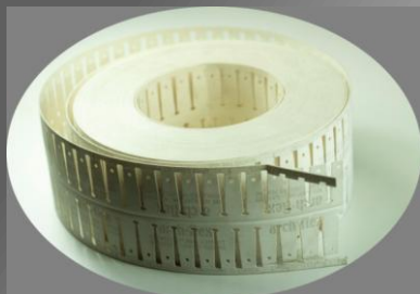
PARASPIGOLO FLESSIBILE IN CARTA AD ANGOLO VARIABILE PER ARCHI Dim. 35x35mm in rotolo da ml 30,5 Codice: NAF13005R
